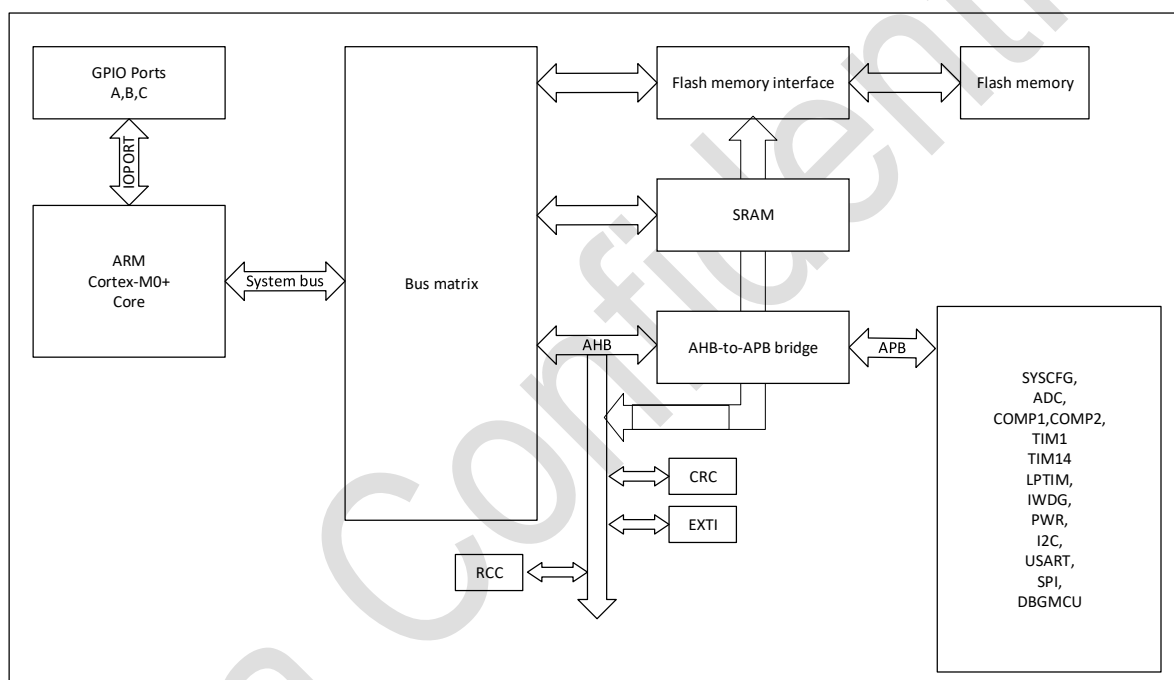
图 3-1 系统架构
