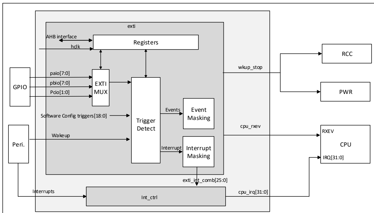
图 11-1 EXTI 框图
