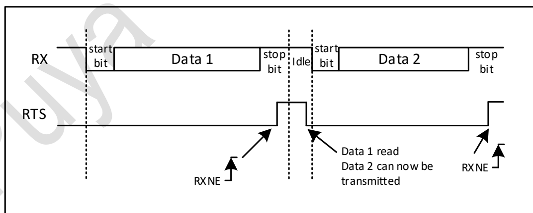
图 20-14 RTS 流控制
