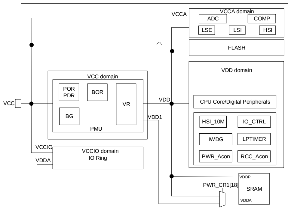
图 5-1 电源框图
