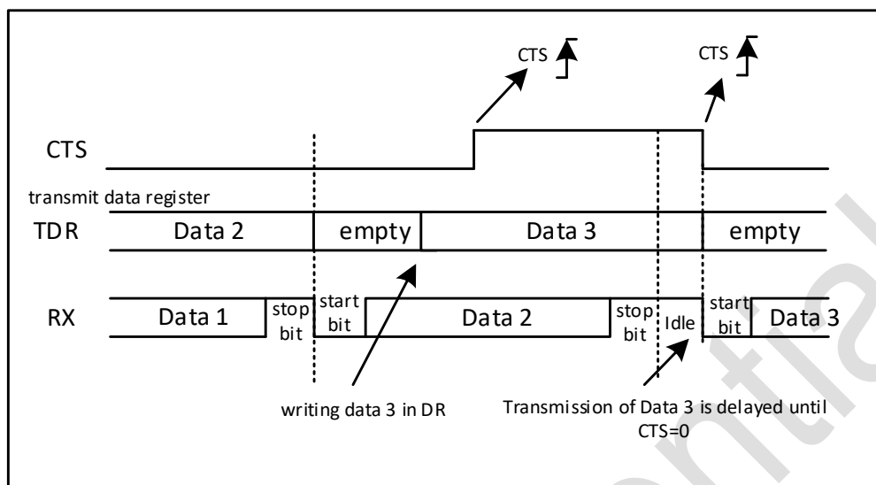
图 20-15 CTS 流控制
