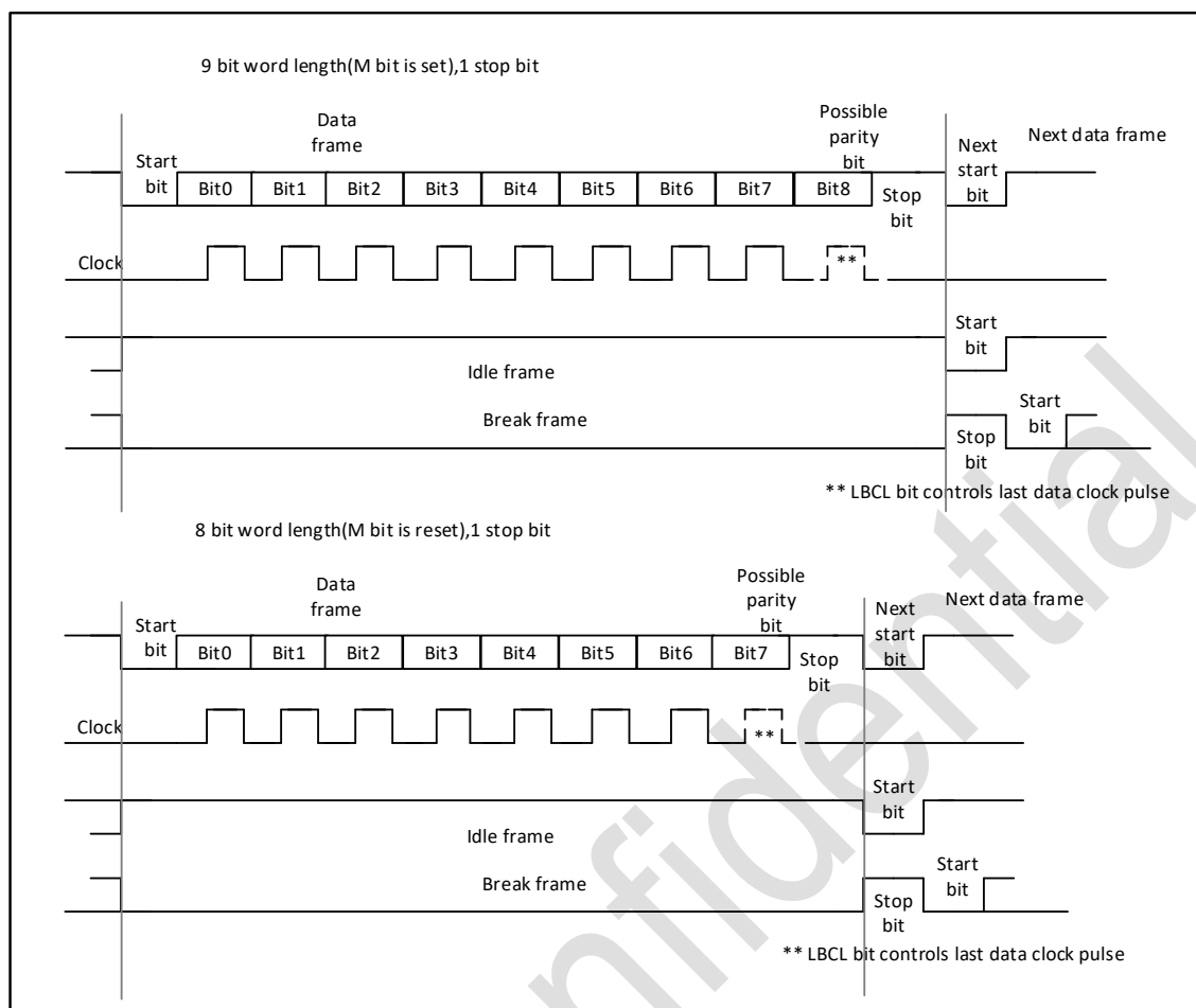
图 20-2 字长设置
