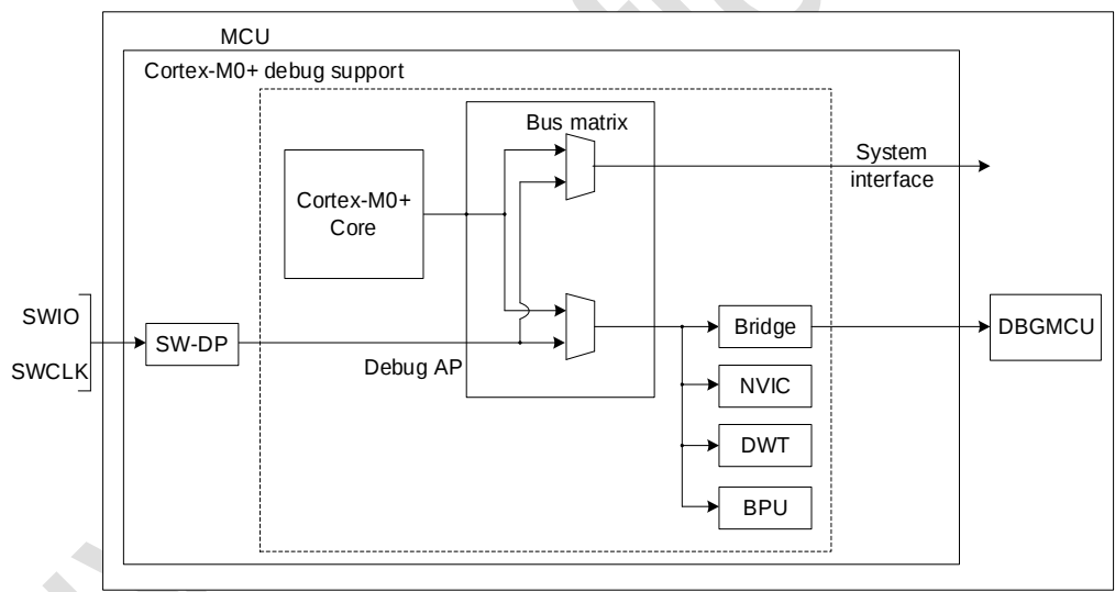
图 22-1 DBG 框图
