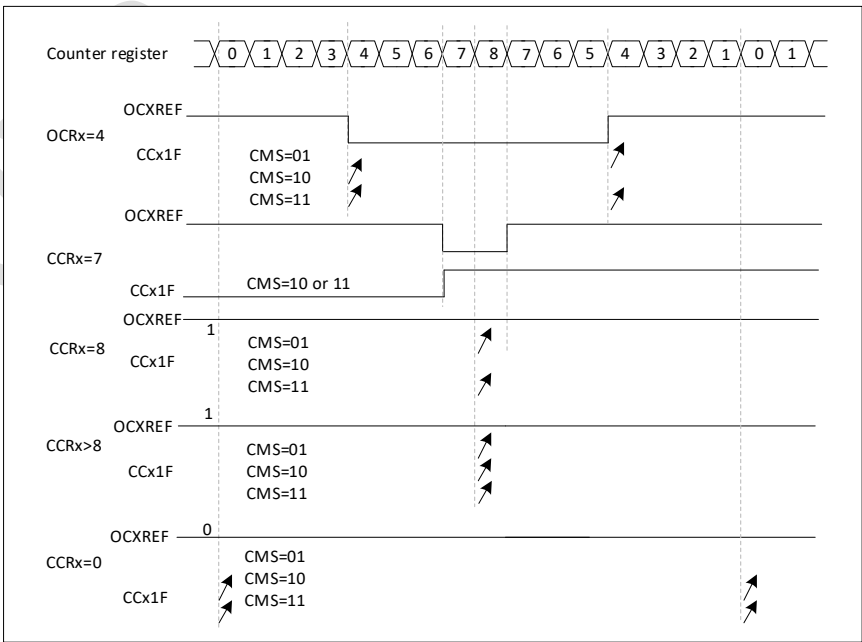
图 15-34 中央对齐的 PWM 波形(APR=8)
