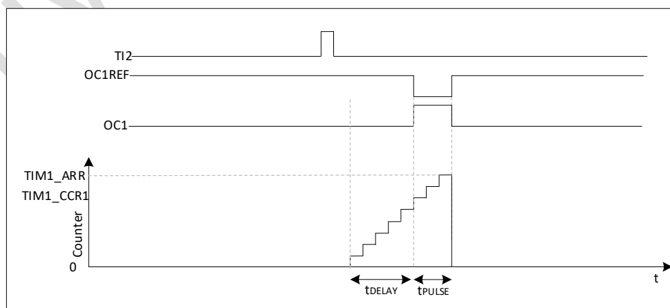
图 16-14 单脉冲模式波形
