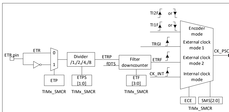
图 15-25 T12 外部触发输入框图
